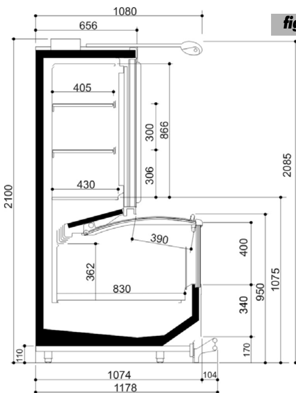
COLISUEM 4 ECO H2000
