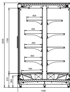
NordicStar MD3 e-Visio 30-148-221
