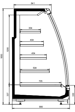
NordicStar SV5 30-99-165
