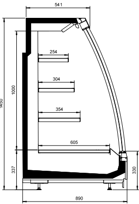
NordicStar SV5 30-89-145
