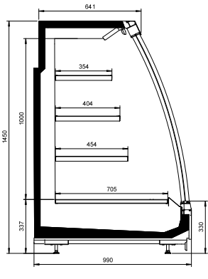
NordicStar SV5 30-99-145
