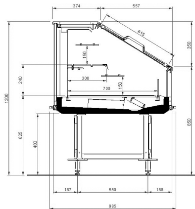
Sezione Stage SV Closed N H12
