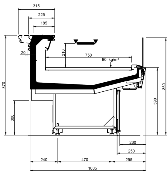
Sezione Velvet C Studio LS-D
