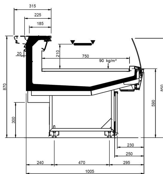
Sezione Velvet C Studio LS-C
