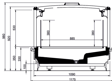
Sezione GranOntario_C
