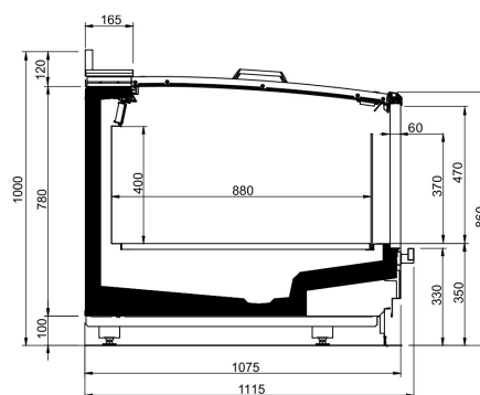
Sezione GranOntario L_GranDrake_EOL_Sliding Covers
